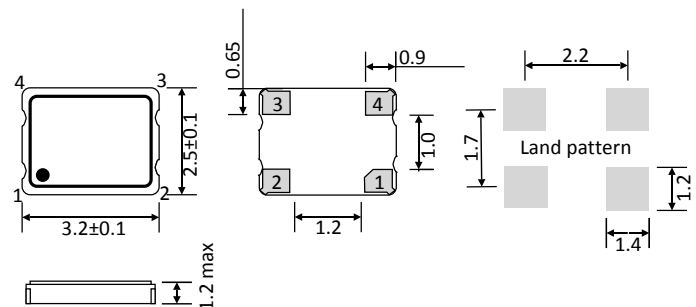
Dimensions(Unit:mm)
