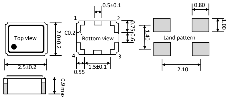
Dimensions(Unit:mm)
